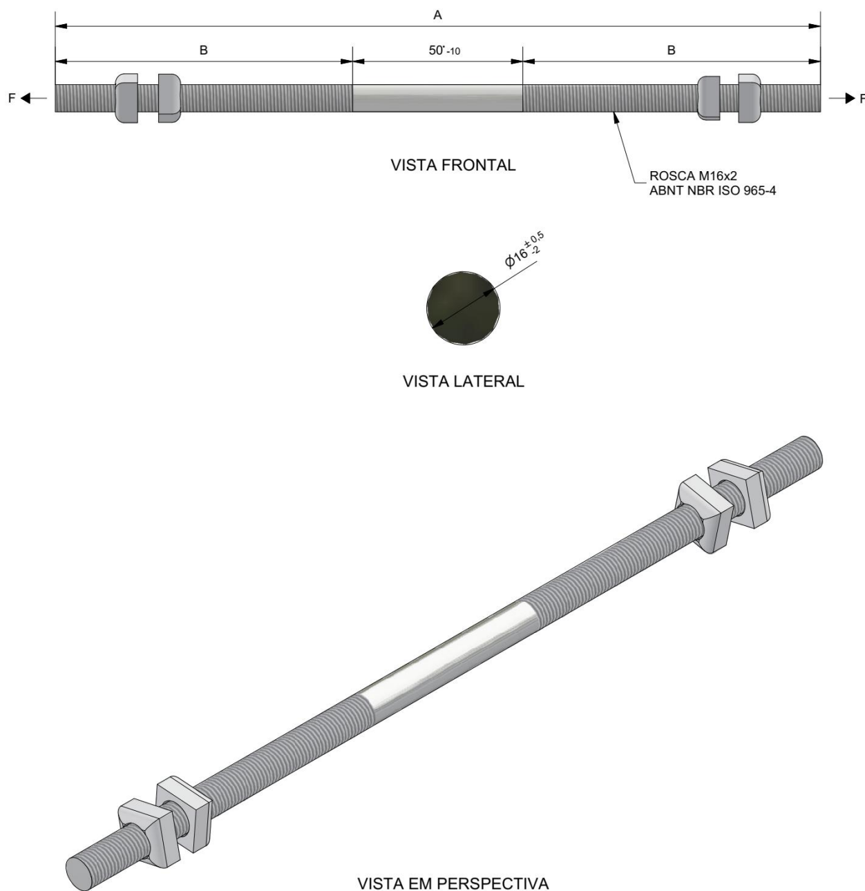
Figura 1 - Parafuso rosca dupla em Liga de alumínio
